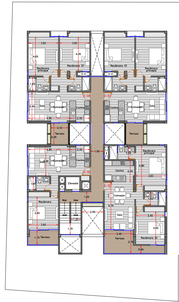
PRIMER NIVEL
