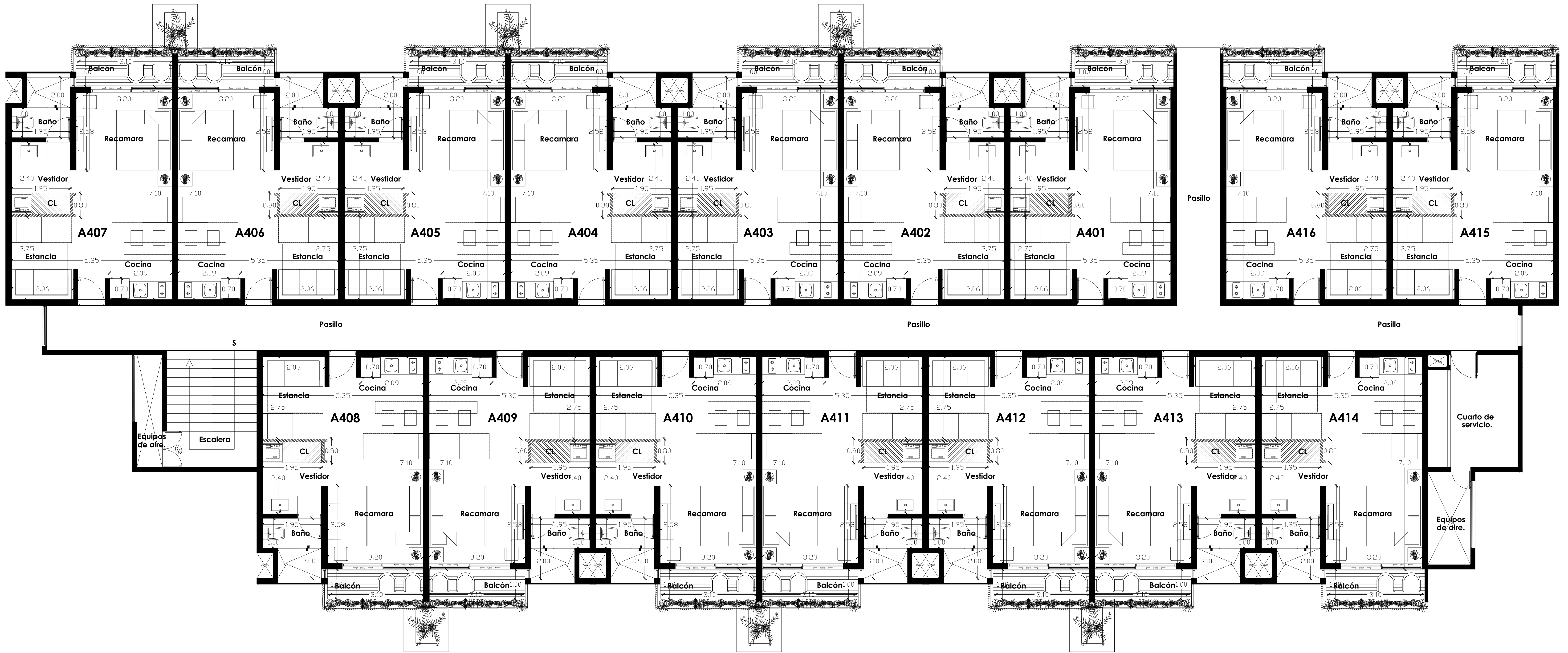
PLANTA CUARTO NIVEL A401-A416
