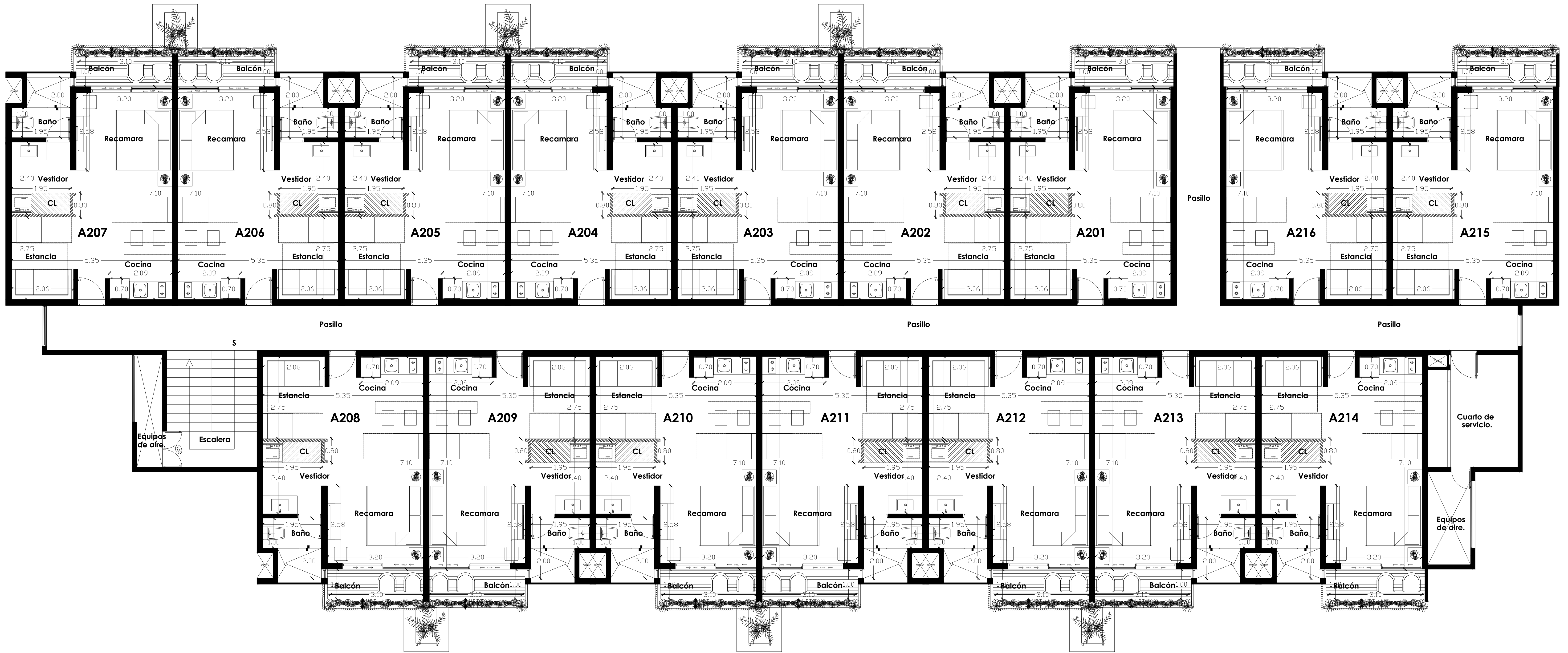
PLANTA SEGUNDO NIVEL A201-A216
