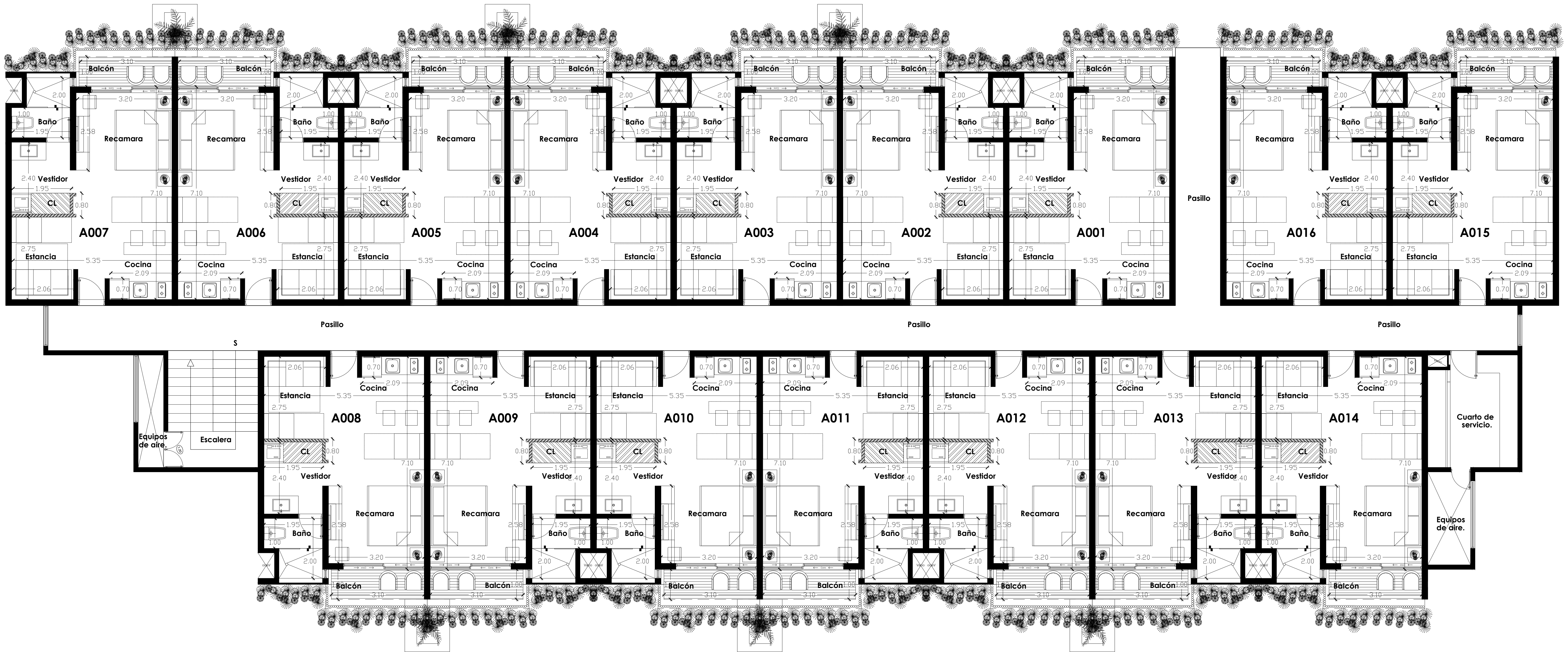
PLANTA BAJA A001-A016
