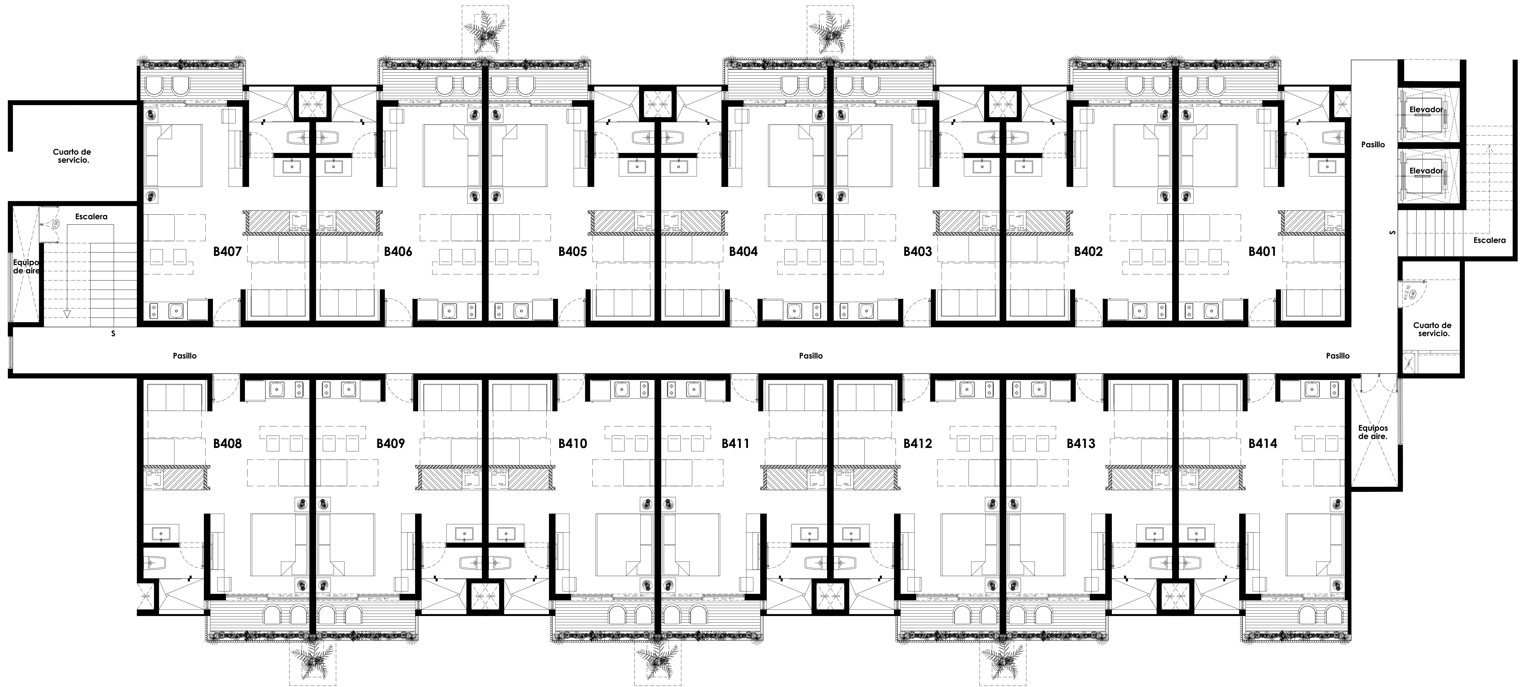
PLANTA CUARTO NIVEL B401-B414
