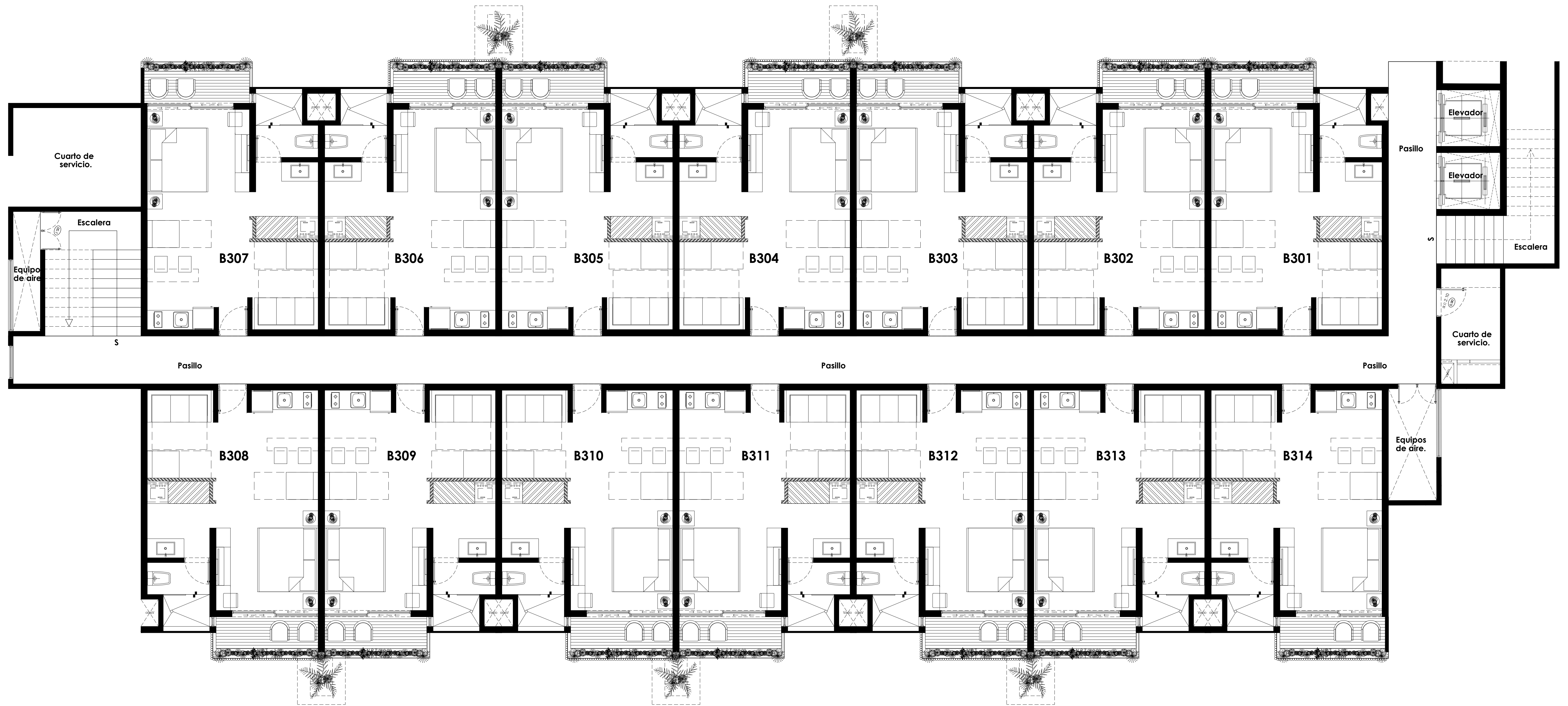
PLANTA TERCER NIVEL B301-B314
