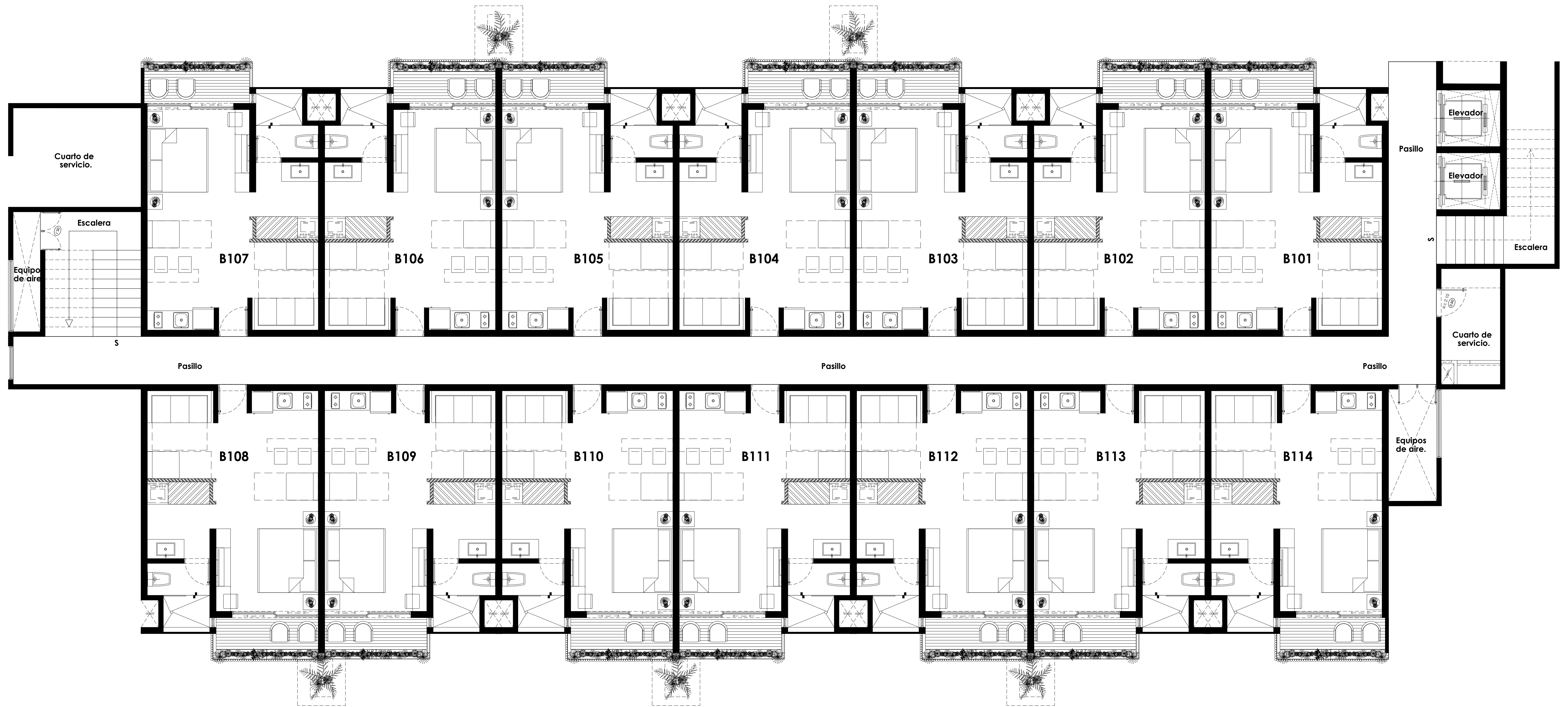
PLANTA PRIMER NIVEL B101-B114
